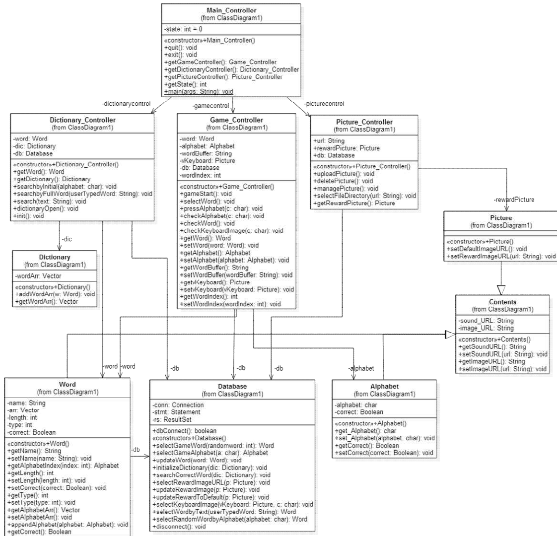
[ 그림 20 ] Class Diagram
